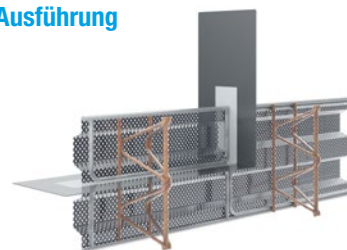
Typ V = verstärkte Ausführung
