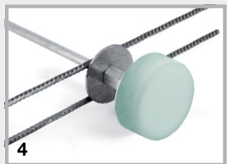
4 Fertig montiert
