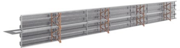
DICHTBLECH Abschalelemente ABS verzahnt – Typ V
